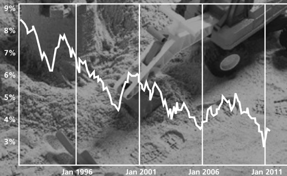
Baugeld-Index (15 Jahre)
